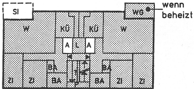
Vollgeschoss / Erdgeschoss
