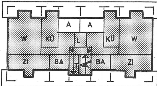
Dachgeschoss Variante 1
