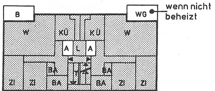
Vollgeschoss / Obergeschoss
